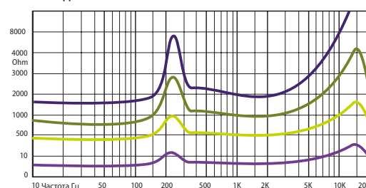
ИМПЕДАНС
